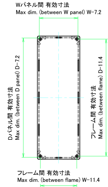
下カバー / Bottom cover
